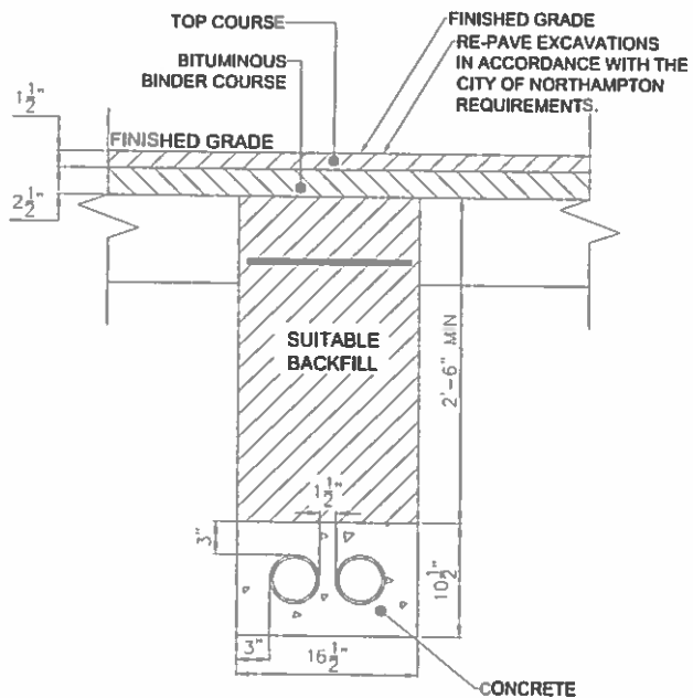
DETAIL A 2-4" DUCTS SCALE: N.T.S
